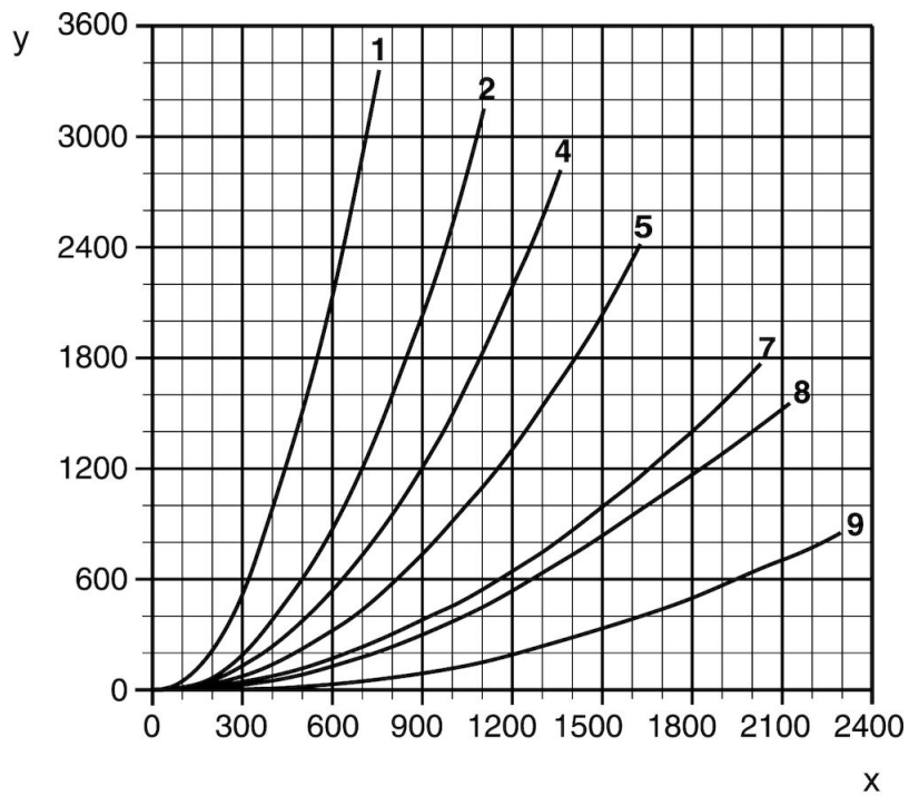
1: Slang diam 75 mm, Längd 5 m; 2: Slang diam 100 mm, Längd 7,5 m; 4: Slang diam 100 mm, Längd 5 m; 5: Slang diam 150 mm, Längd 7,5 m; 7: Slang diam 150 mm, Längd 6 m; 8: Slang diam 150 mm, Längd 5 m; 9: Slang diam 200 mm, Längd 6 m
