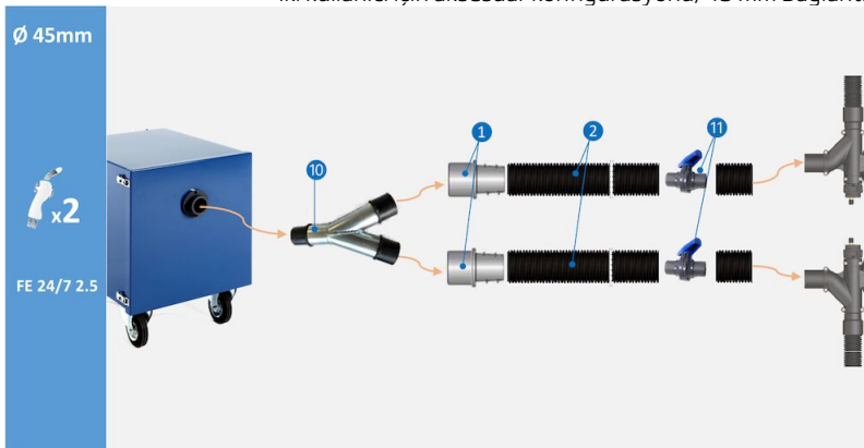
İki kullanıcı için aksesuar konfigürasyonu, 45 mm Bağlantı:
