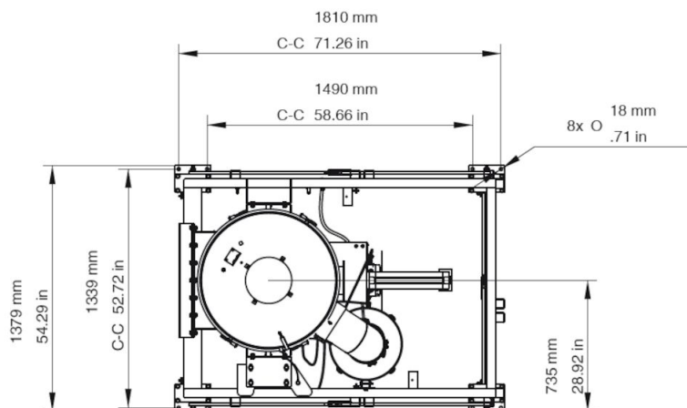
FlexFilter Single Vysoké provedení
