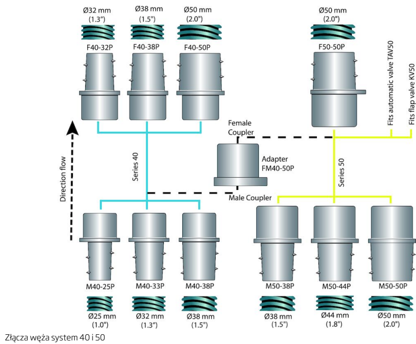
Złącza węży system 40 i 50
